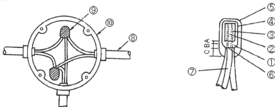
線心接続部
