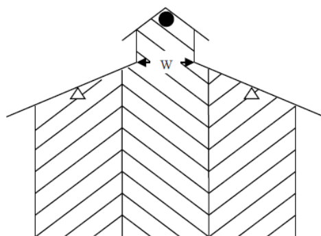
第 25-102 図 (断面図)
