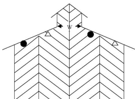
第 25-103 図 (断面図)
