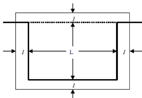
第 25-64 図 一边省略の例 2
