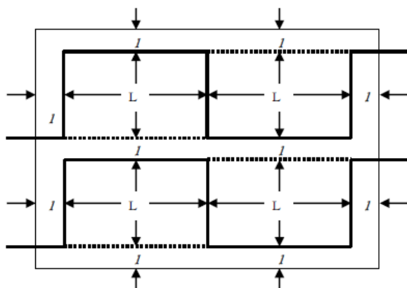
第 25-65 図 二辺省略の例 1
