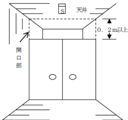
第 25-61 図 (立面図)
