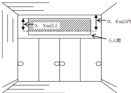
第 25-47 図 (立面図)
