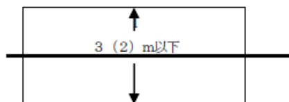
第 25-67 図 一边省略と二辺省略の組合せの例 1
