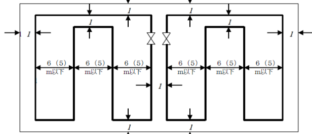
第 25-68 図 一边省略と二边省略の組合せの例 2 (特に広い居室の場合)
