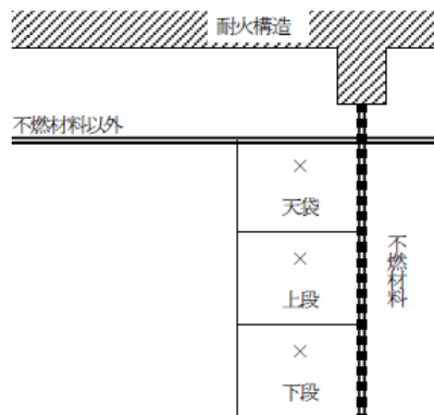
(ウ) 押入等の壁が不燃材料のもの 第 25-14 図
