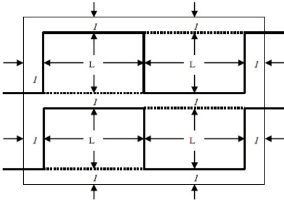
第 25-65 図 二辺省略の例 1
