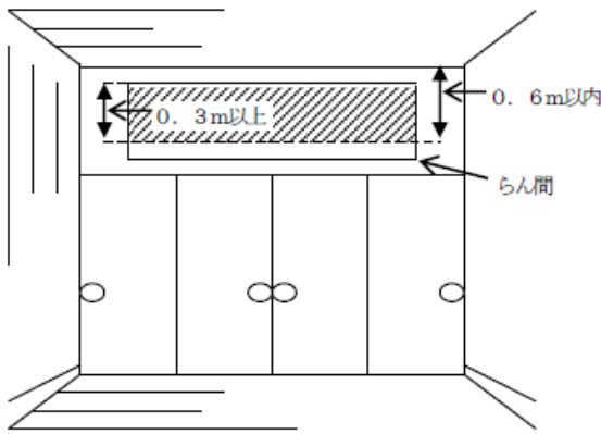
第 25-47 図 (立面図)
