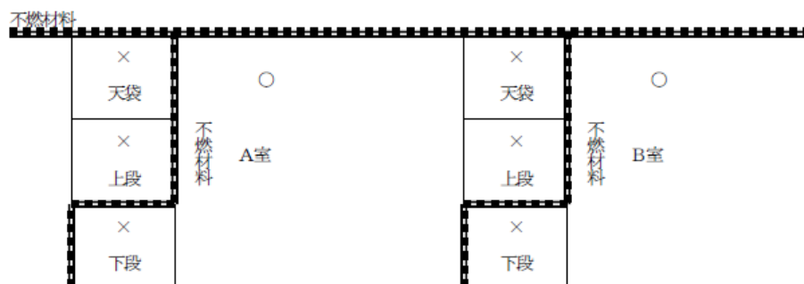
(イ) 押入等の壁及び天井が不燃材料以外のもの 第 25-17 図
