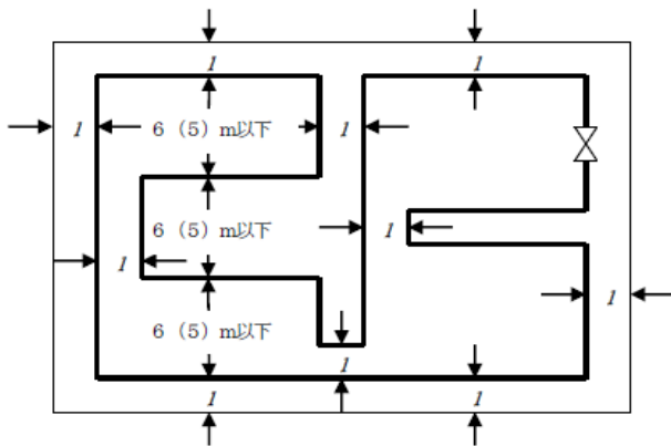
第 25-67 図 一辺省略と二辺省略の組合せの例 1
