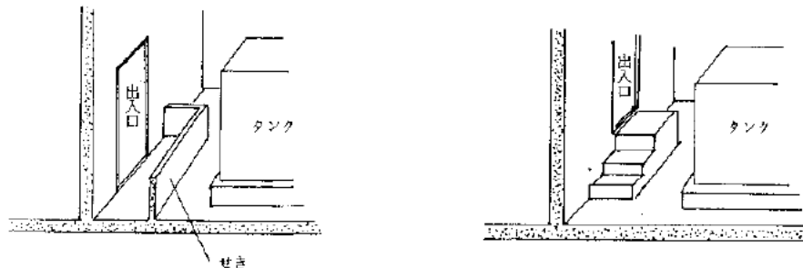
階層設置の屋内タンク貯蔵所の参考例
