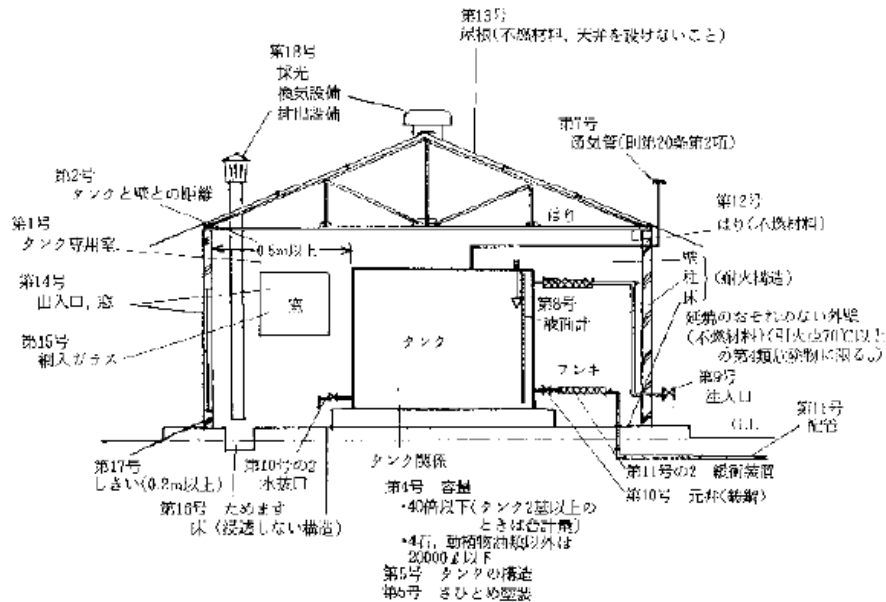
図 屋内タンク貯蔵所参考例
