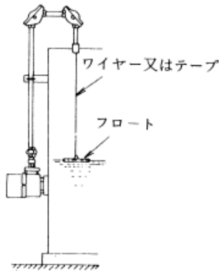
図 浮子式計量装置の例
