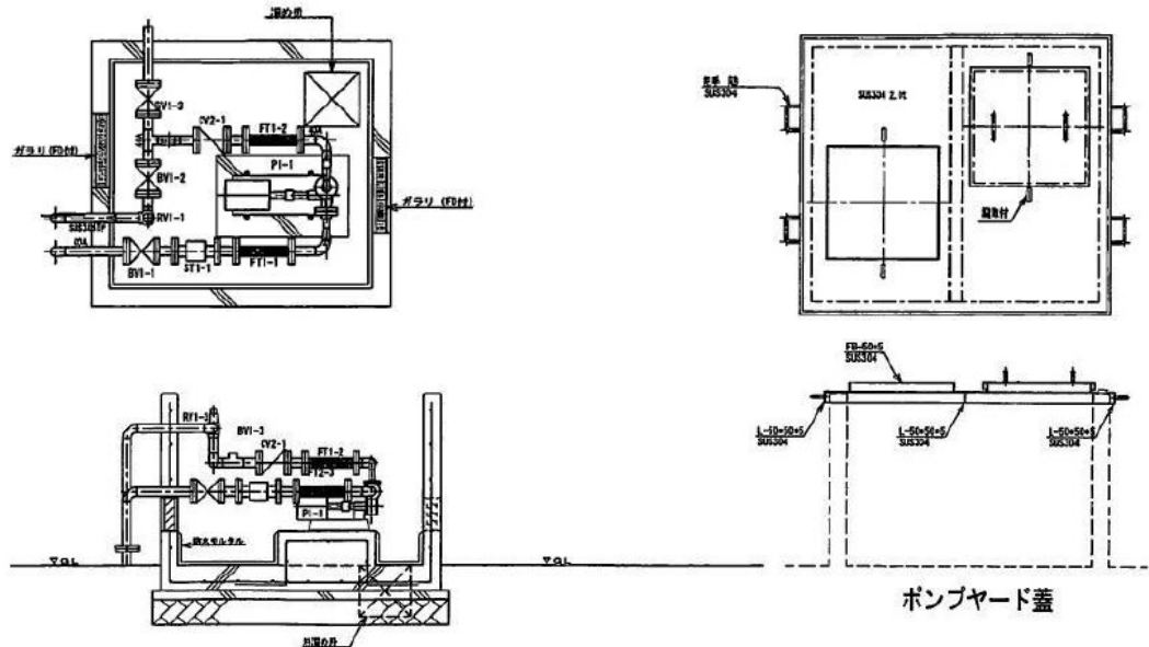
図 人が中に入ることができない小さなポンプ室の例
