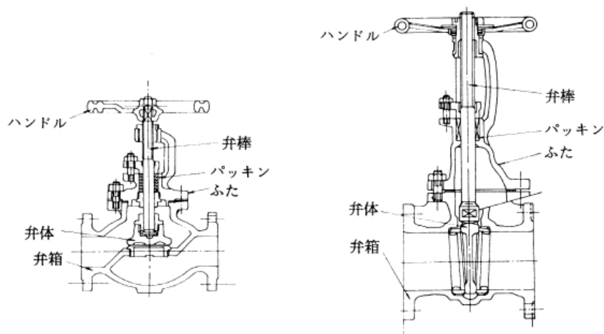
図 玉形弁の例
