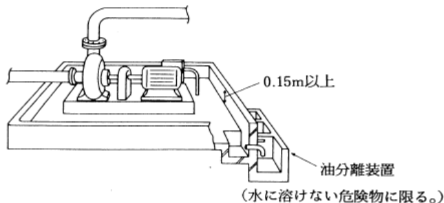
図 屋外のポンプ設備の例
