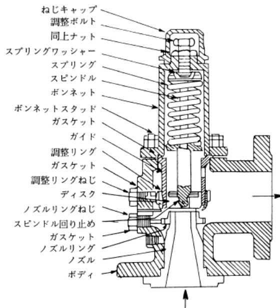
図 安全弁の構造例
