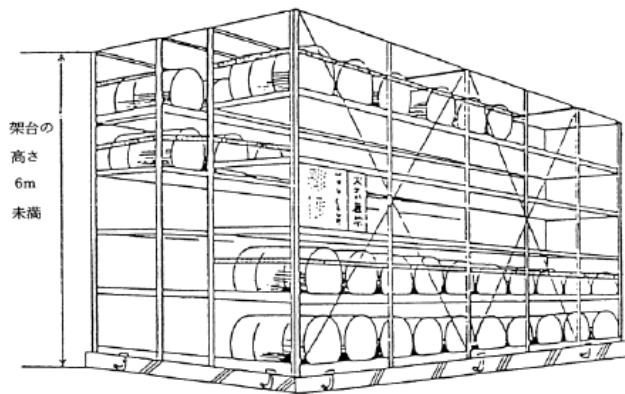
図 架台の高さ
