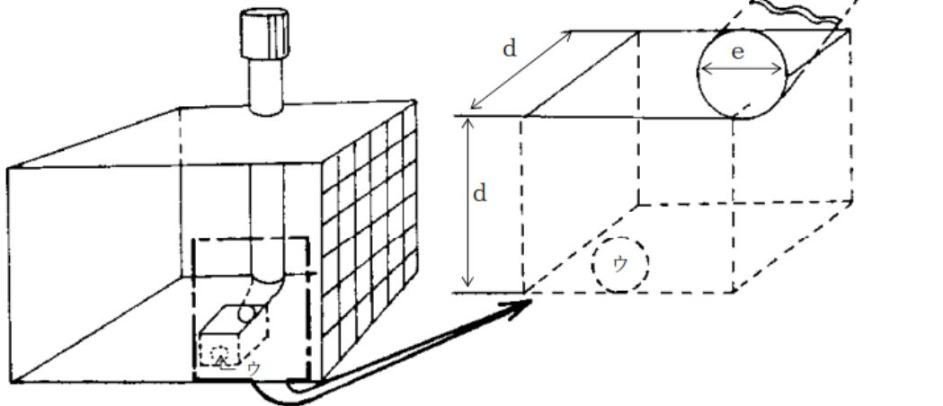
例図2 ーためますを整備室の中央に設ける場合の例ー
