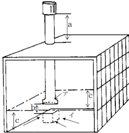
例図1 ーためますを整備室の隅に設ける場合の例ー
