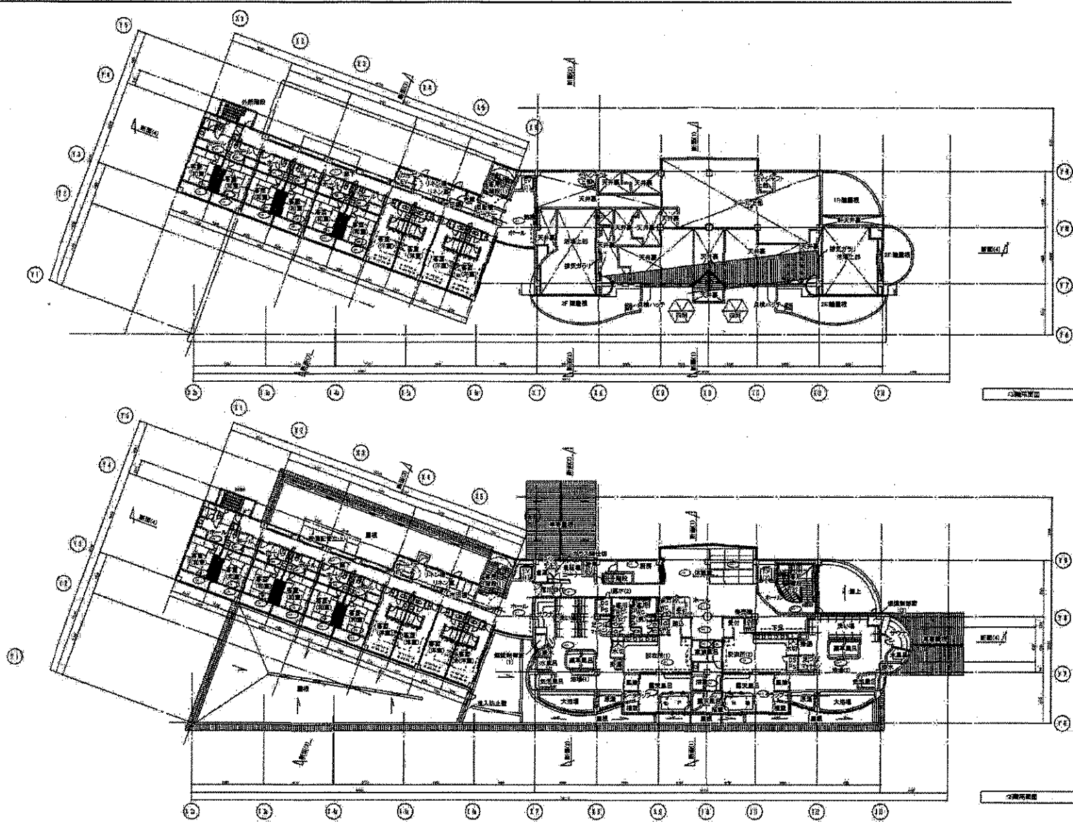
44 白浜町健康交流拠点施設「リヴァージュ・ジュース」 55 2階・3階 平面図
